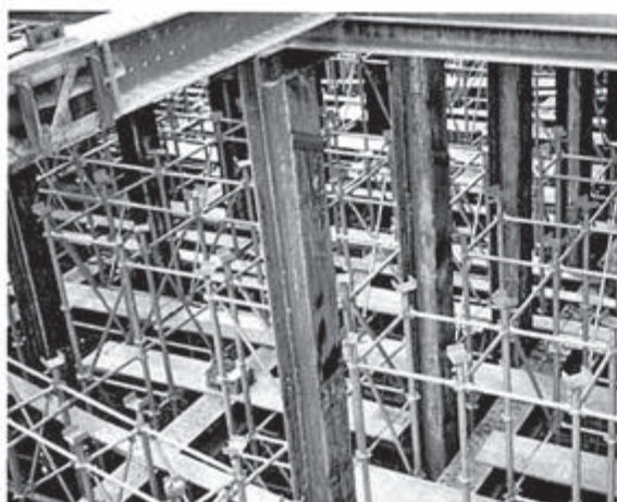
■JR地下駅舎
