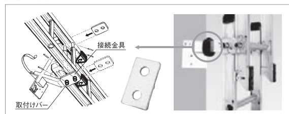
接続金具
